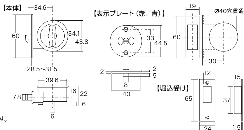
バックセット 30mm 適用扉厚 28mm ~ 35mm
